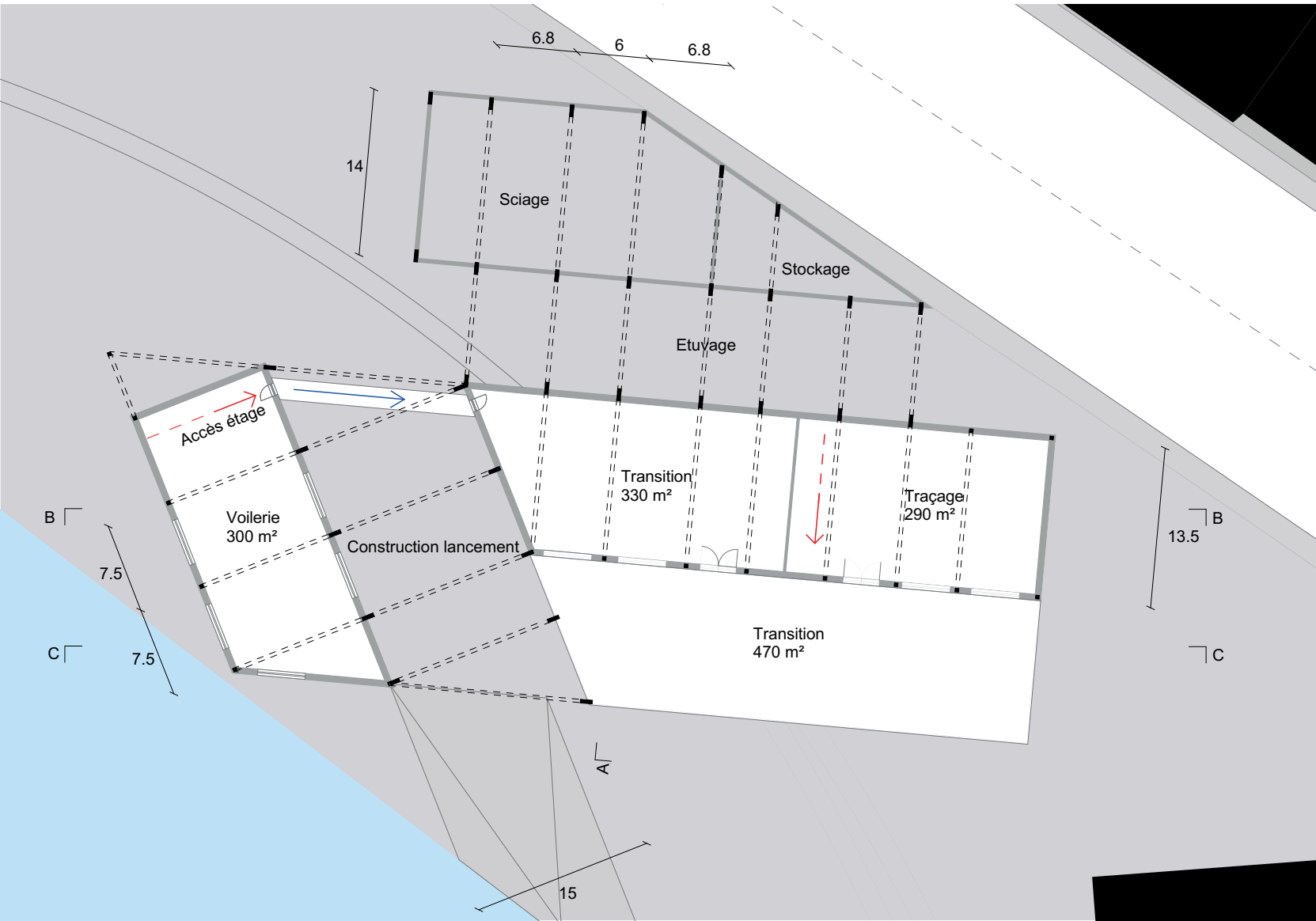
PLAN D'ESQUISSE R+1 1:500 EME
