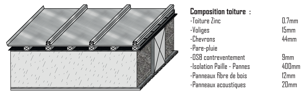
AXONOMETRIE DETAIL TOITURE ISOLEE 1:20 EME
