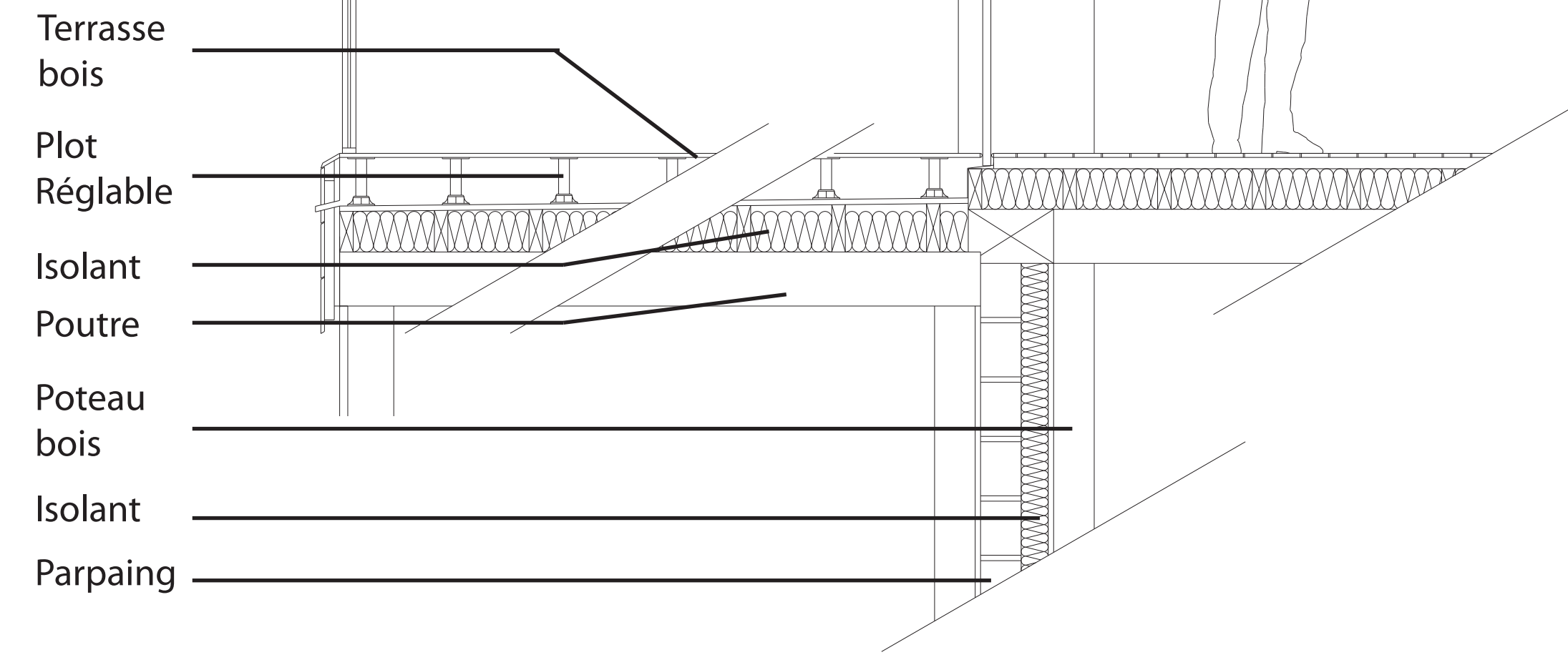
Détail technique extension 1/20 0 0.5 1
