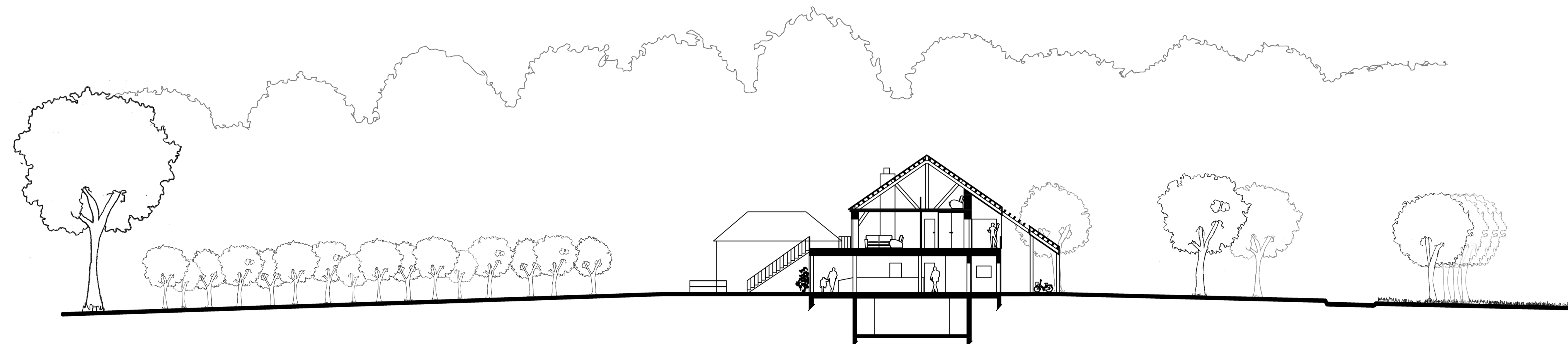
Coupe transversale magasin 1/200 0 5 10m
