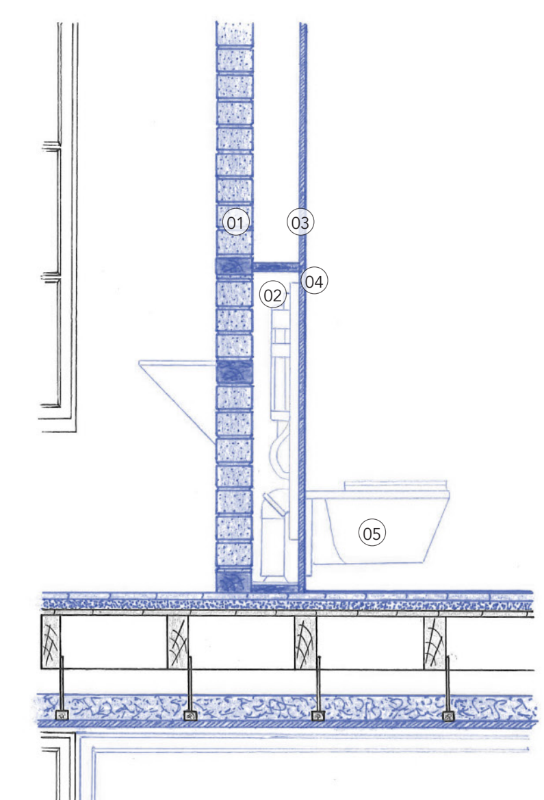
DÉTAIL 03 Ech. : 1/20 ème
