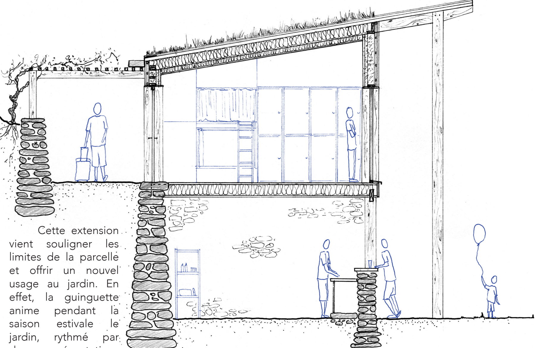
COUPE A - EXTENSION GUINGUETTE Ech. : 1/50 ème
