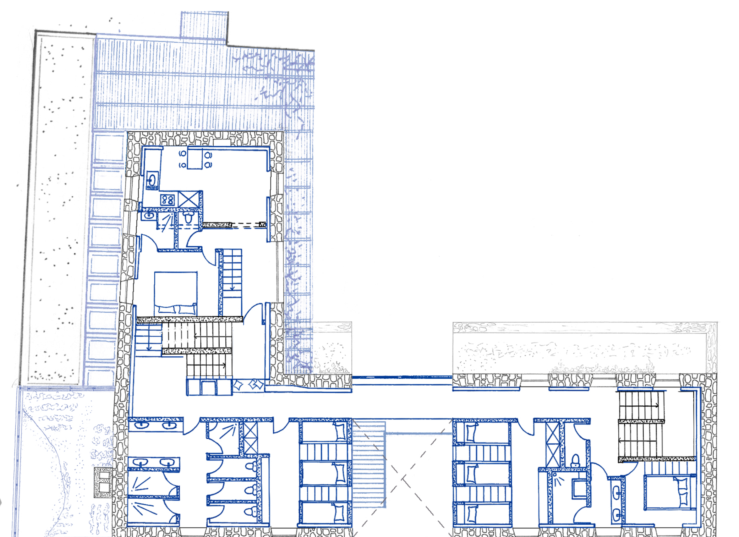
N PLAN R+1 PROJET Ech. : 1/100 ème
