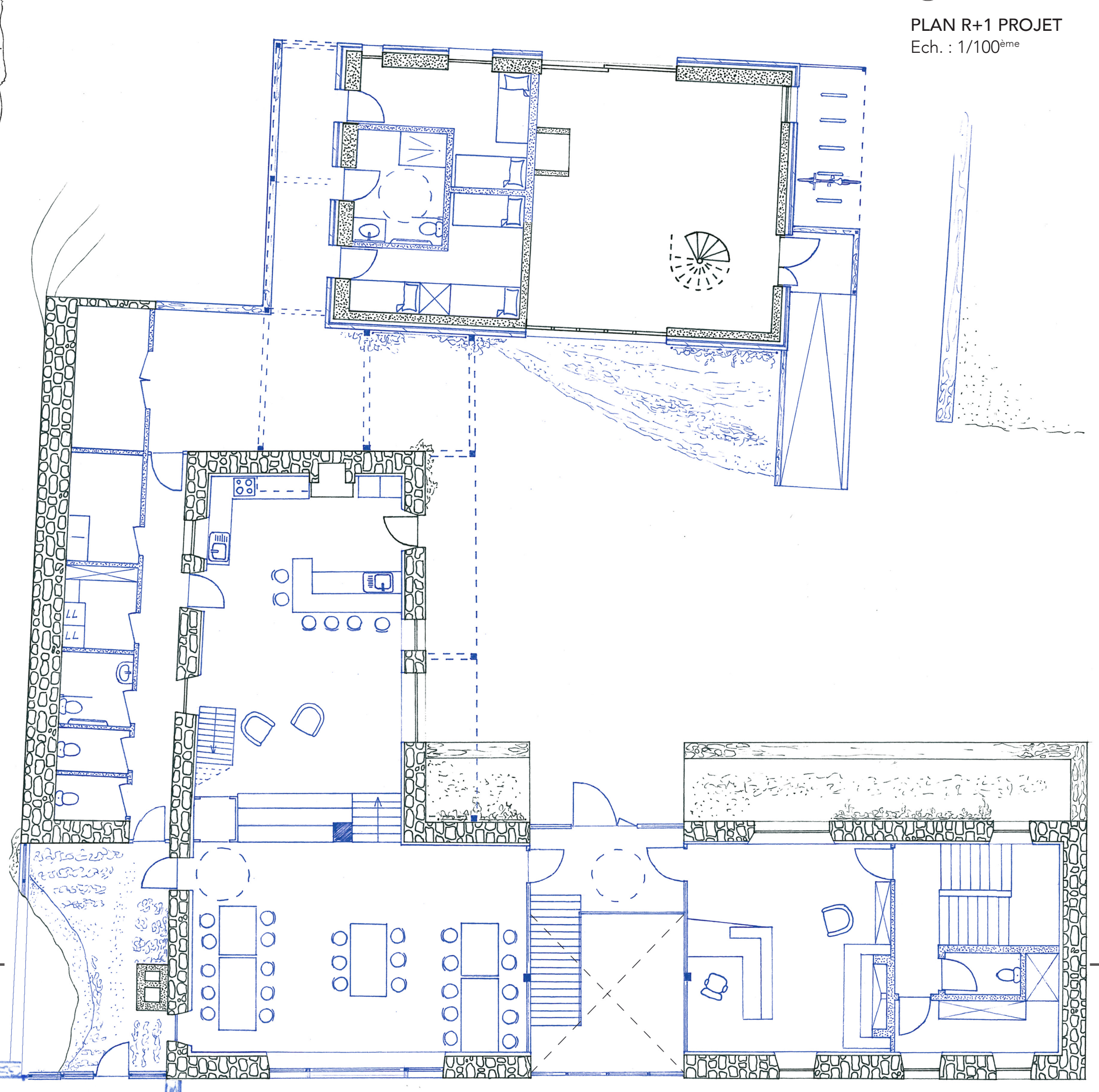
N PLAN RDC PROJET Ech. : 1/100 ème
