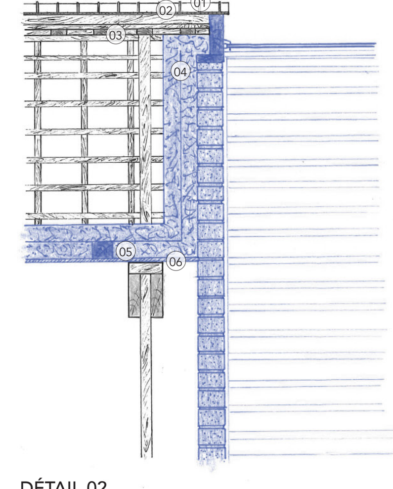
DÉTAIL 02 Ech. : 1/20 ème
